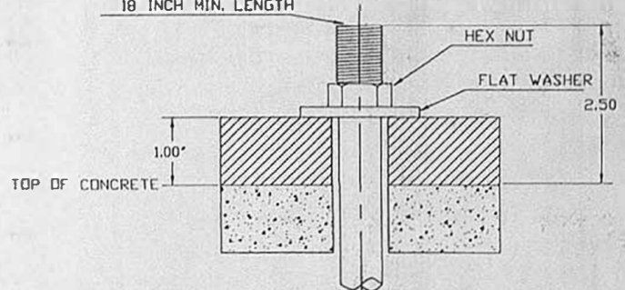
ANCHOR BOLT PROJECTION SCALE: N.T.S.
